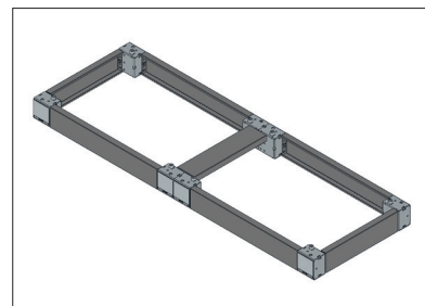
Configurazione per passaggio cavi sotto la flangia orizzontale
