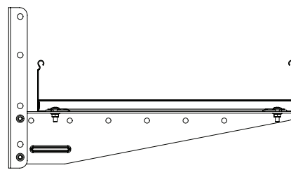
Montaggio della passerella a scaletta su mensola rivettata Ladder mounting to riveted bracket
