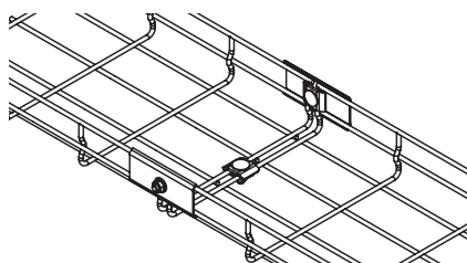
Piastrina di accoppiamento lineare Flat coupler
