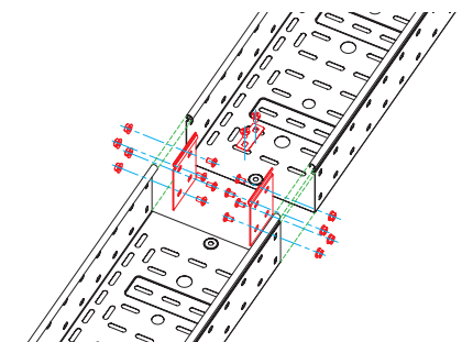
Giunzione tramite giunto lineare - h 100 mm Joint with flat coupler - h 100 mm
