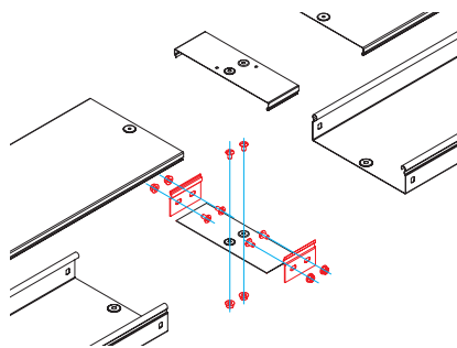
Coprigiunto base e coprigiunto coperchio Splice plates for width and cover
