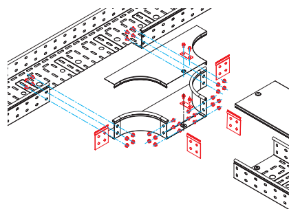
Derivazione a T laterale Side tee
