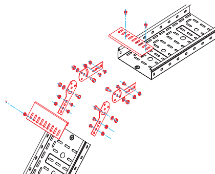
Ribordo di protezione con giunti a snodo verticali Protection plate and vertical adjustable couplers
