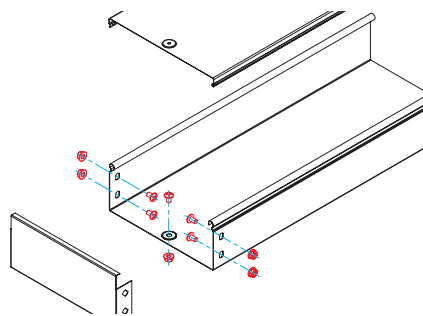
Testata di chiusura h 80 mm Stop end - 80 mm
