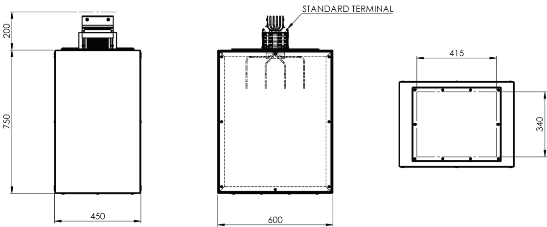
DIMENSIONI ALIMENTAZIONE - B160 / B200 / B240 END FEEDER DIMENSIONS - B160 / B200 / B240
