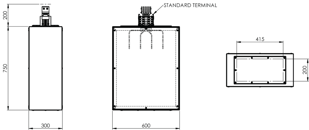
DIMENSIONI ALIMENTAZIONE - B60 / B80 / B100 END FEEDER DIMENSIONS - B60 / B80 / B100
