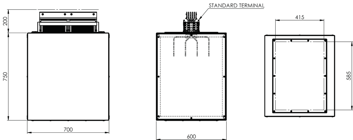
DIMENSIONI ALIMENTAZIONE - 2B160 / 2B200 / 2B240 END FEEDER DIMENSIONS - 2B160 / 2B200 / 2B240
