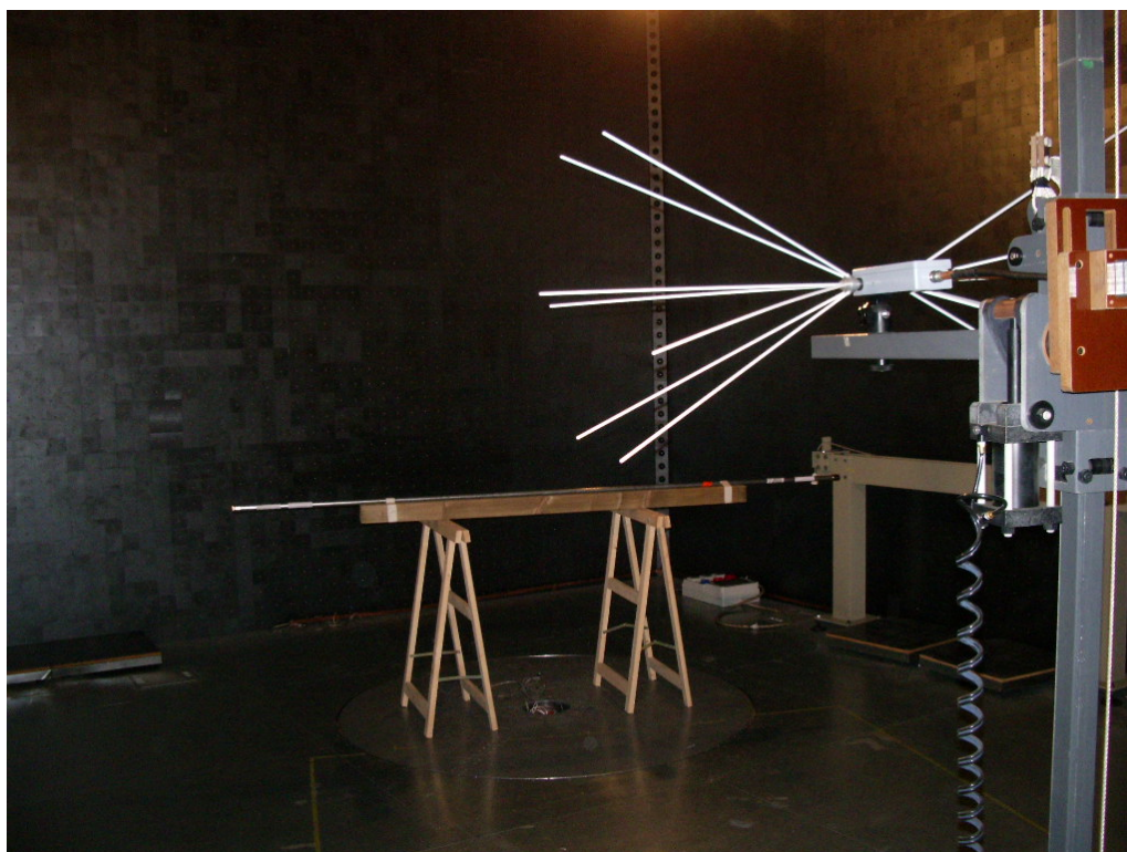
Tubo rigido acciaio zincato in camera schermata semi-anecoica.
